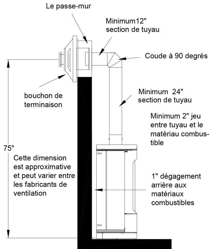
Figure 4 - Configuration de ventilation minimum et dégagements
