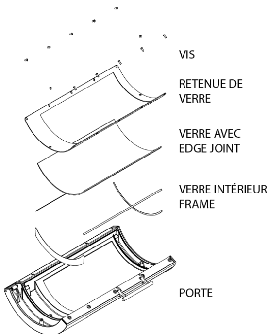
Figure 4: L'assemblage de la porte
