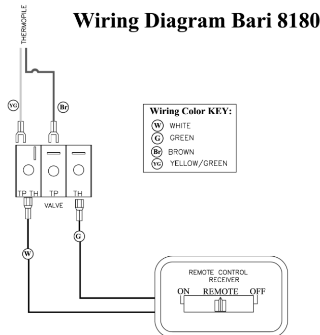
Figure 10: Bari DV 8180 Schéma de câblage
