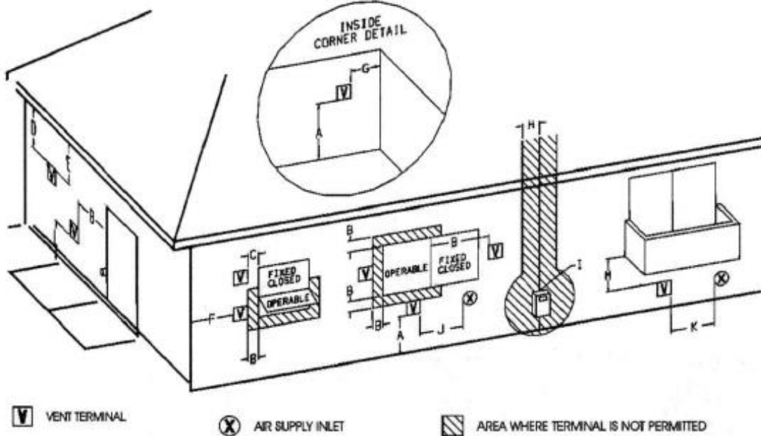
Figure 5: Emplacement acceptable de la Terminaison
