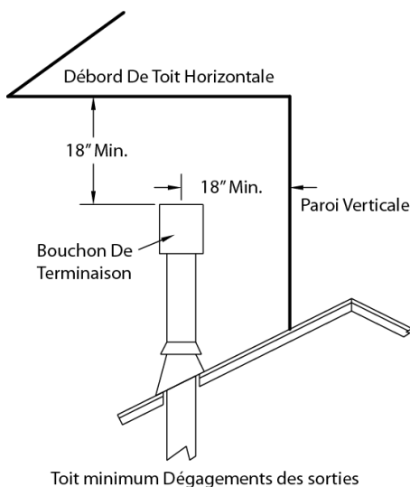
Figure 9 : Dégagements de Cap de terminaison
