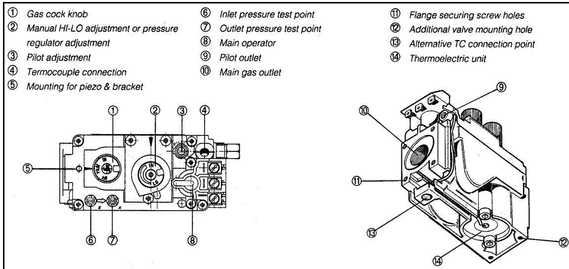
Figure 11: Valve de Contrôle du Gaz
