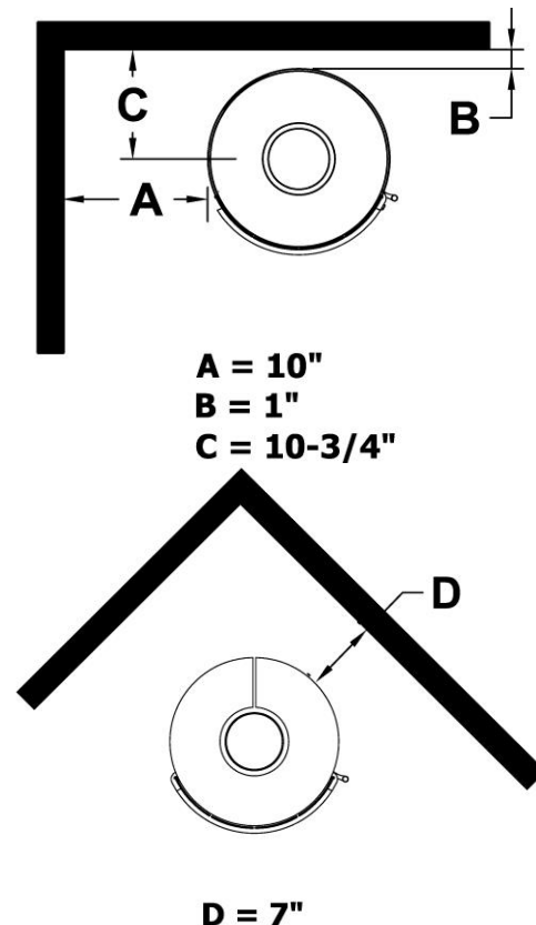
Figure 2 – 8180 Minimum Dégagements
