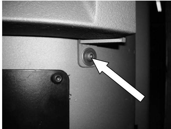
Figure 3 – Enlever la vis pour l'accès Firebox
