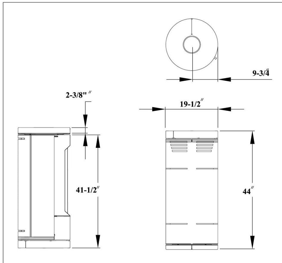
Figure 1 – Dimensions du Modèle 8180 (en pouces)
